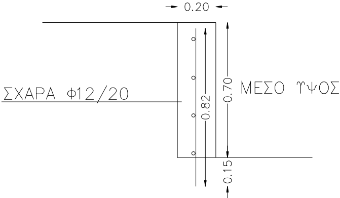
ΤΜΗΜΑ 2 & 4 ΤΟΜΗ ΤΟΙΧΙΟΥ ΚΛΙΜΑΚΑ 1:20
