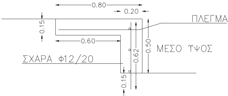
ΤΜΗΜΑ 1 ΤΟΜΗ ΤΟΙΧΙΟΥ ΚΛΙΜΑΚΑ 1:20
