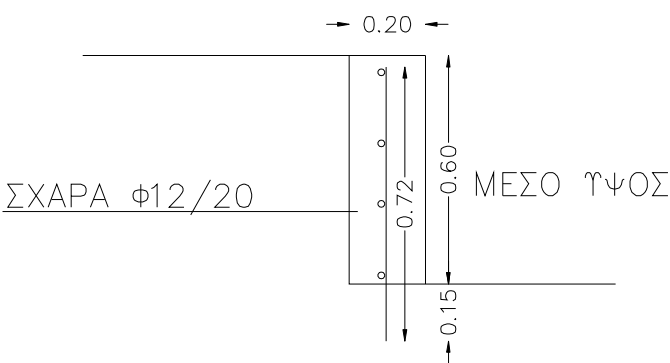
ΤΜΗΜΑ 3 & 5 ΤΟΜΗ ΤΟΙΧΙΟΥ ΚΛΙΜΑΚΑ 1:20
